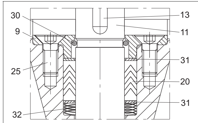
Fig. 17 Gland packing
