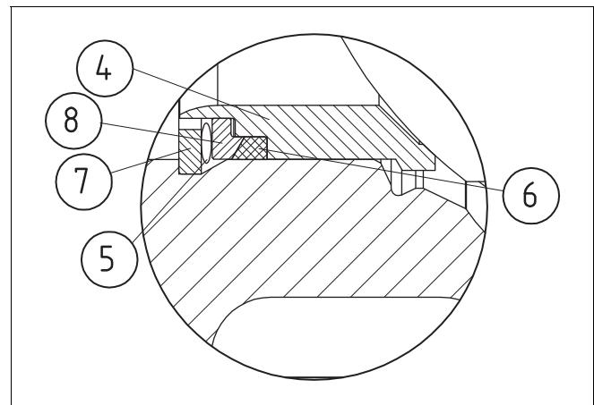
Fig. 34 A-seat
